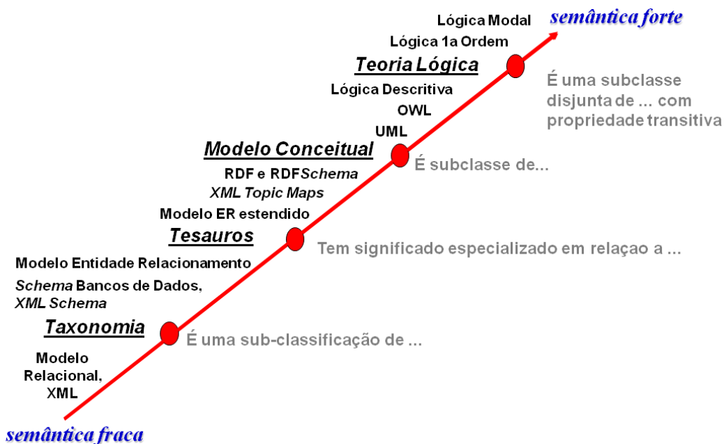
Figura 6: espectro analisado
